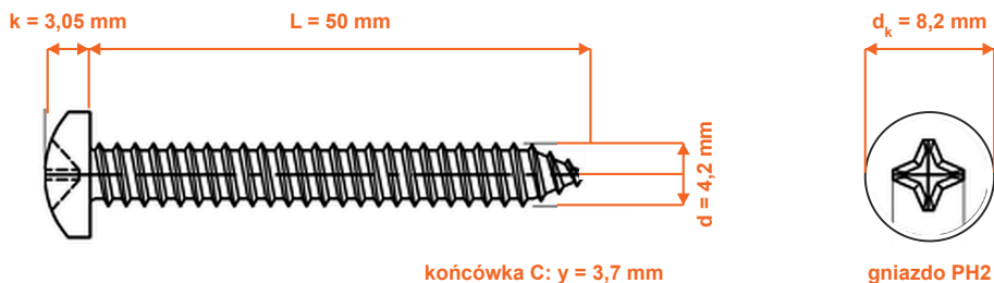
Rysunek poglądowy · DIN 7981 · wartości w mm
