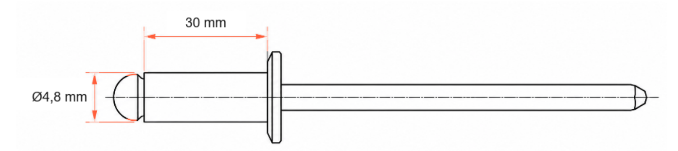
Schemat poglądowy. Wymiary w mm; wartości graniczne podano w tabeli.
