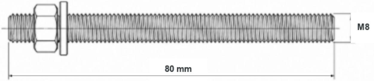
Schemat poglądowy. Wymiary w mm; geometria zakończeń może zależeć od partii produktu.
