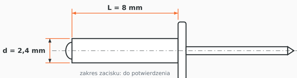
Rysunek poglądowy, bez zachowania skali. Wymiary w mm dla tego produktu.
