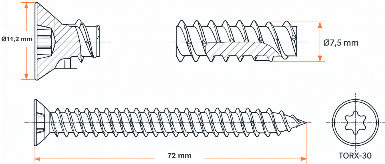
Rysunek poglądowy. Wymiary w mm.
