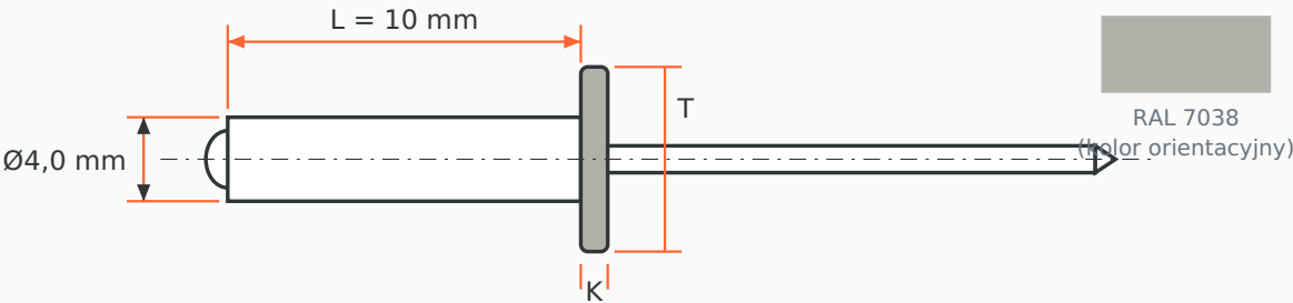
Schemat poglądowy, bez zachowania skali. Wymiary w mm; wartości graniczne podano w tabeli.
