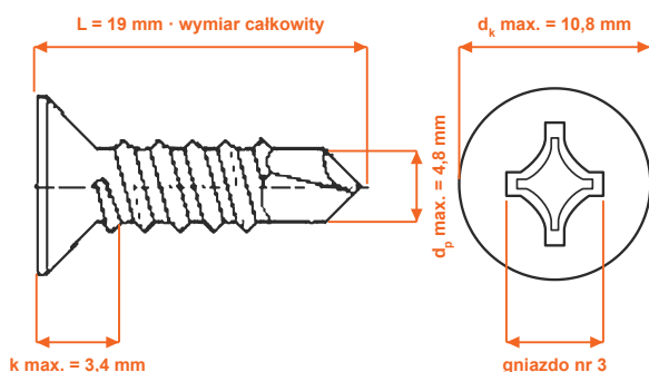
Rysunek poglądowy · DIN 7504 O · d_p max. 4,8 mm · blacha 1,75–5,25 mm · wartości w mm
