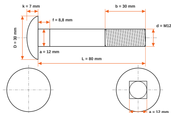
Wymiary wg DIN 603 - wartości w mm
