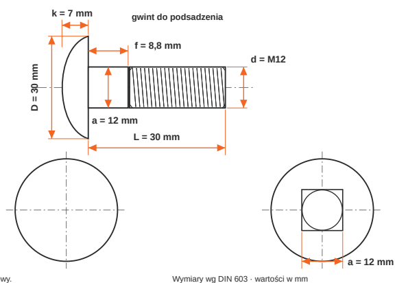
Wymiary wg DIN 603 - wartości w mm
