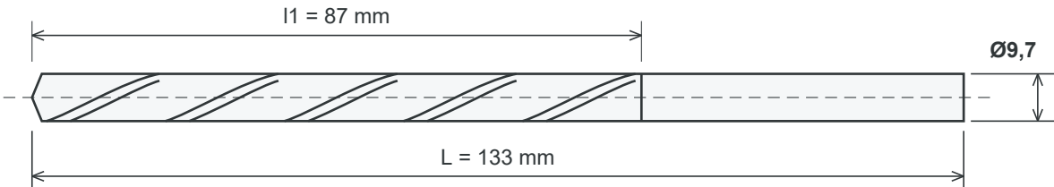
Schemat poglądowy. Wymiary w mm. Kąt wierzchołkowy: 135°.
