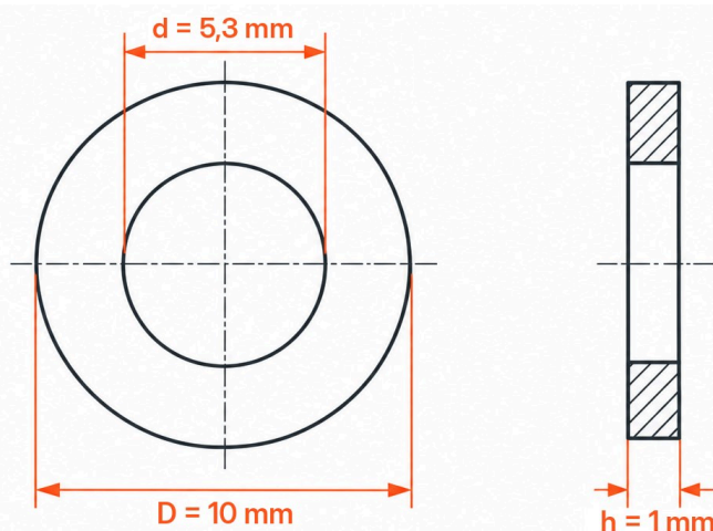
Wymiary wg DIN 125 · wartości w mm
