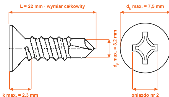
Rysunek poglądowy · DIN 7504 O · d_p max. 3,2 mm · blacha 0,7–2,4 mm · wartości w mm
