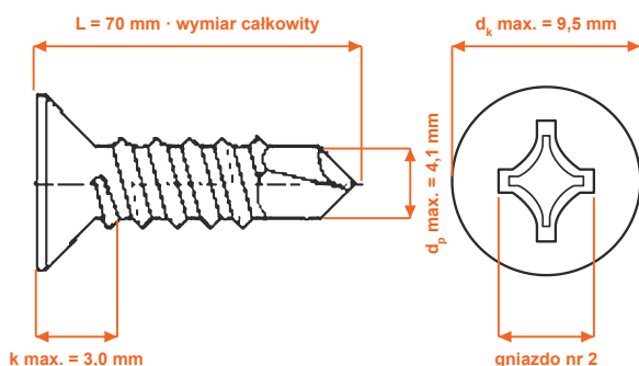
Rysunek poglądowy · DIN 7504 O · d_p max. 4,1 mm · blacha 1,75–4,4 mm · wartości w mm
