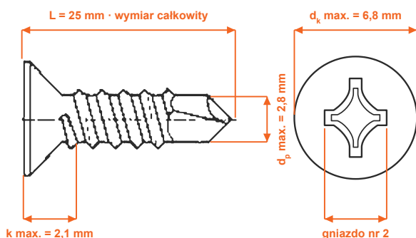
Rysunek poglądowy · DIN 7504 O · d_p max. 2,8 mm · blacha 0,7–2,25 mm · wartości w mm
