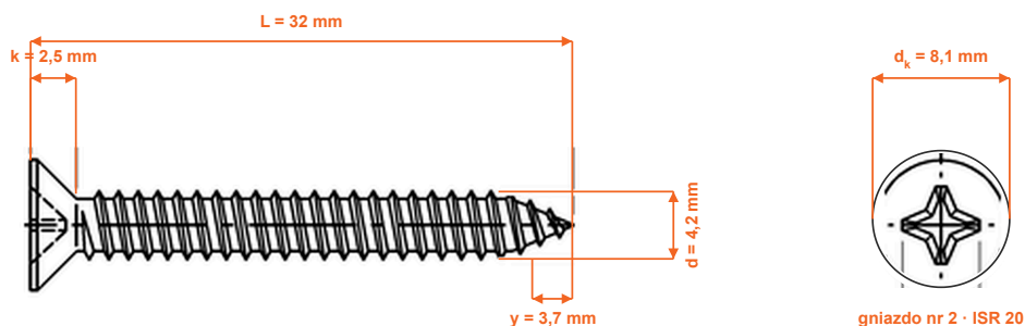
Rysunek poglądowy · DIN 7982 · wartości w mm
