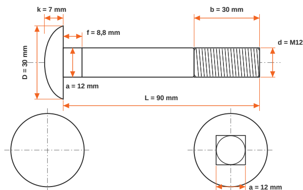
Wymiary wg DIN 603 - wartości w mm
