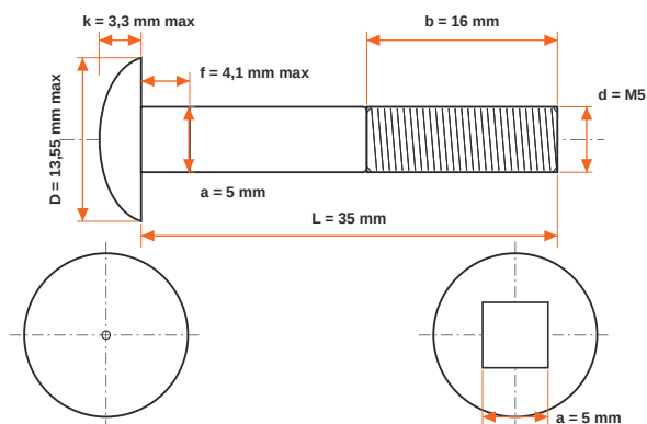
Wymiary wg DIN 603 - wartości w mm
