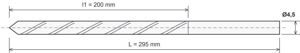
Schemat poglądowy. Wymiary w mm. Kąt ostrzenia: 135°.
