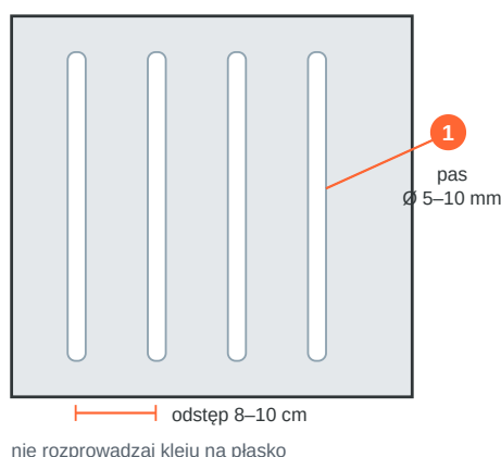
A. TYŁ LUSTRA – PIONOWE PASY KLEJU
